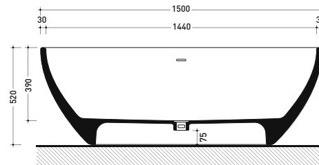
sezione longitudinale / section
